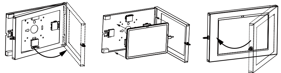
Position Guide
